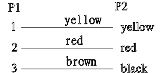
接线示意图
