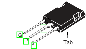
PLUS247 (IXTX)
