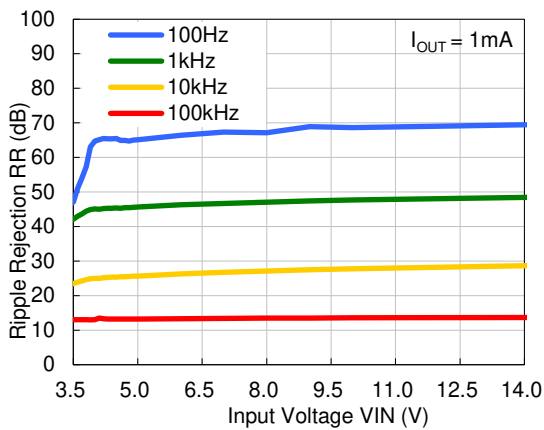
VR=3.3V, I OUT =1mA
