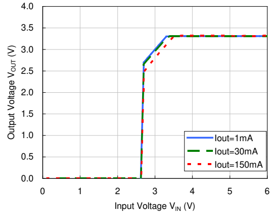
VR=3.3V
