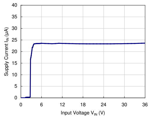
VR=3.3V
