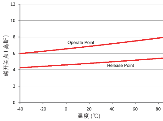
图2. SM351LT的典型性能特点
