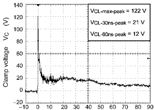
Fig. 6.1.1 +8 kV
