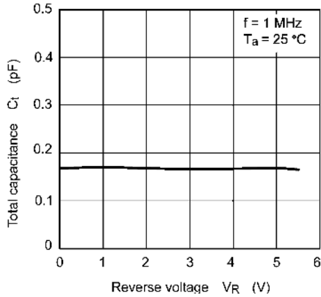
Fig. 9.3 C_t - V_R
