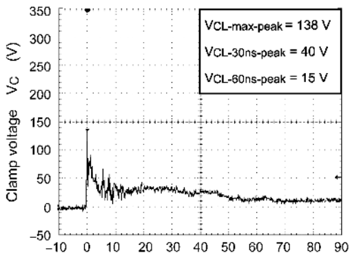
Fig. 6.1.3 +15 kV
