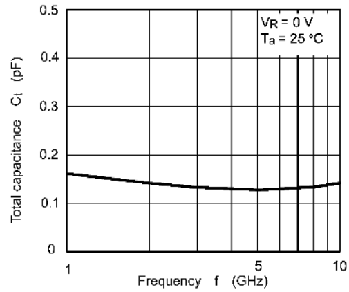
Fig. 9.4 C_t - f
