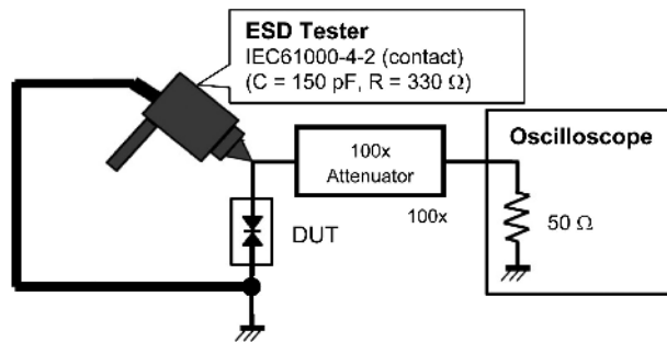
Fig. 6.1.5 IEC61000-4-2 (Contact)
