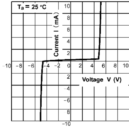
Fig. 9.1 I - V
