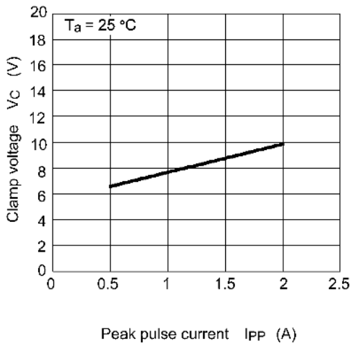
Fig. 6.3.1 V_C - I_{PP}
