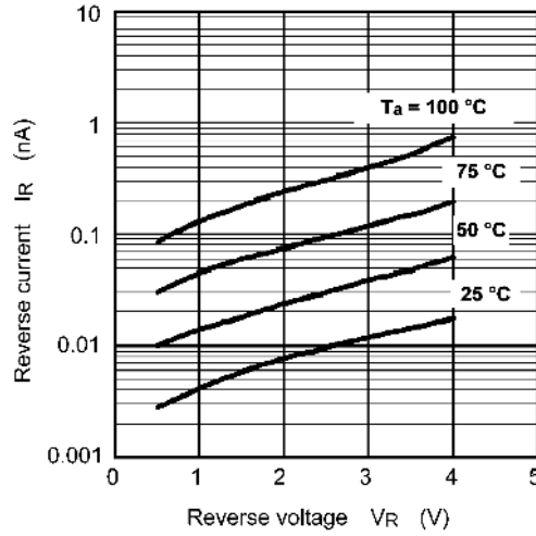
Fig. 9.2 I_R - V_R
