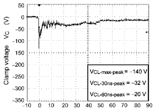
Fig. 6.1.4 -15 kV
