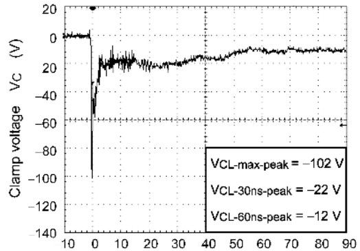
Fig. 6.1.2 -8 kV
