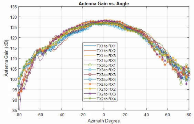
62 – 64 GHz
