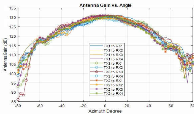
60 – 62 GHz
