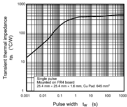
Fig. 8.11 r_{th} - t_w
