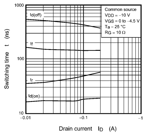
Fig. 8.10 t - I_D
