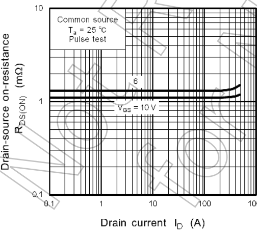
Fig. 9.5 R_{DS(ON)} - I_D
