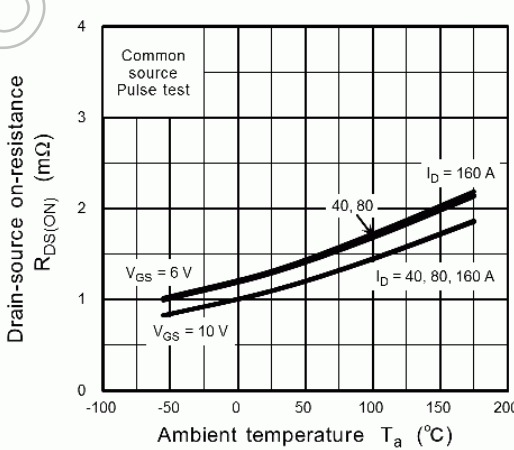
Fig. 9.6 R_{DS(ON)} - T_a
