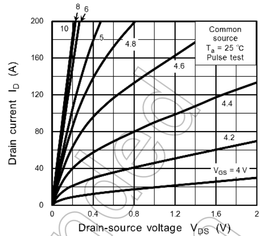
Fig. 9.2 I_D - V_{DS}
