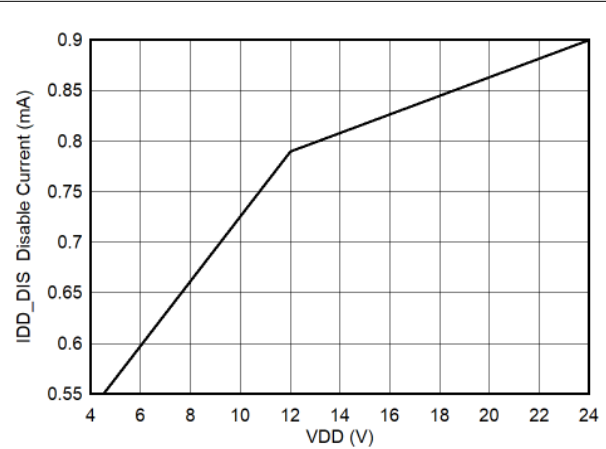
Figure 6-6. Disable Current (EN = 0 V)
