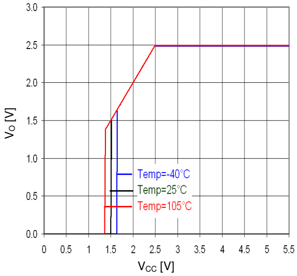
Figure 27. Vcc-Vo (Io=0mA)
