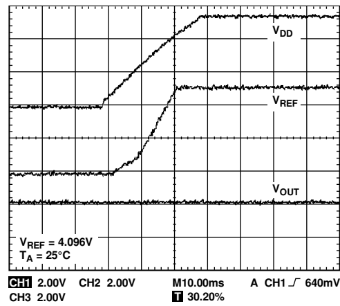
Figure 26. POR to 0V
