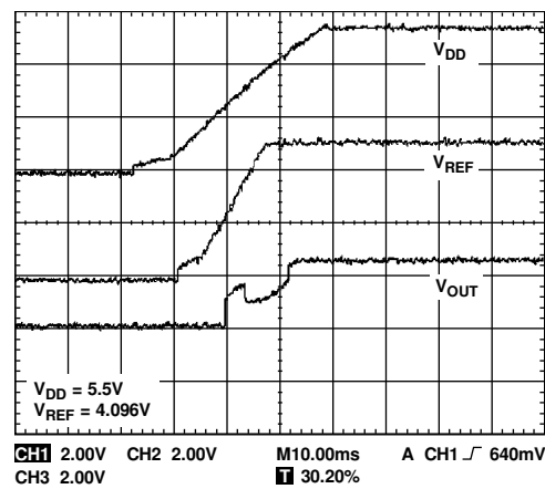
Figure 27. POR to MS
