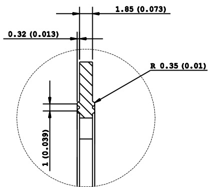
Dettaglio: 1 Scala 3:1
