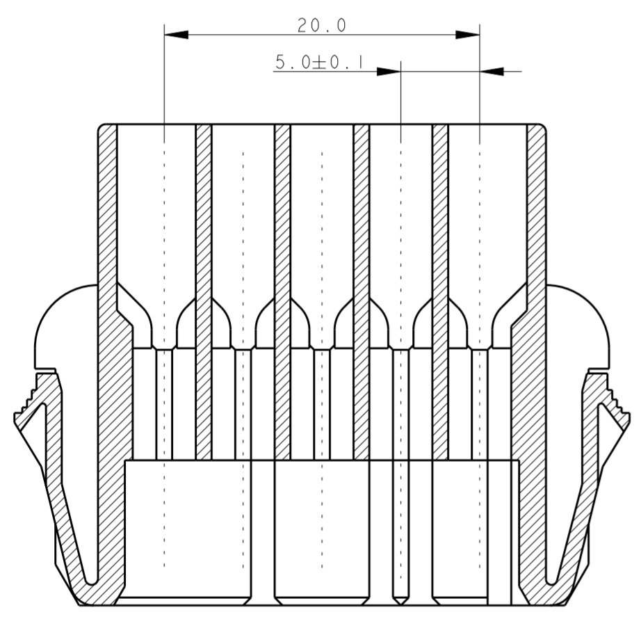
SECTION D-D
