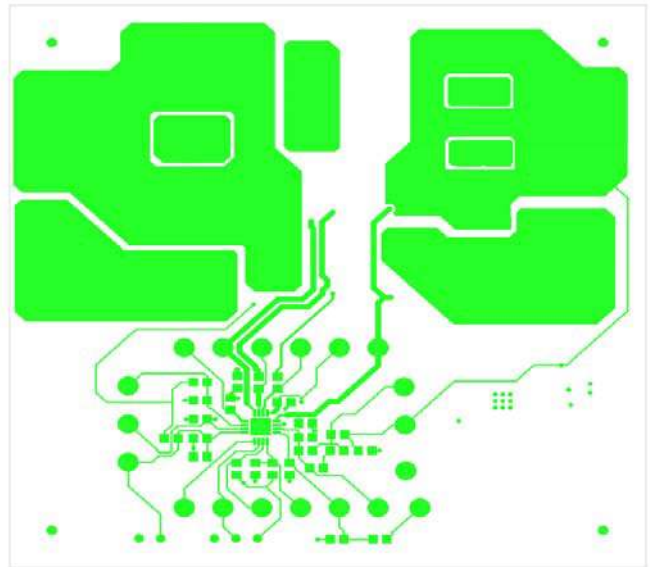
FIGURE 22. TOP LAYER
