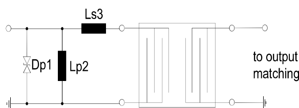
Fig. 2 Suppressor diode plus ESD matching
