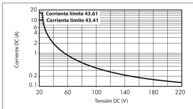
H 43 - Máximo poder de corte con cargas en DC1
