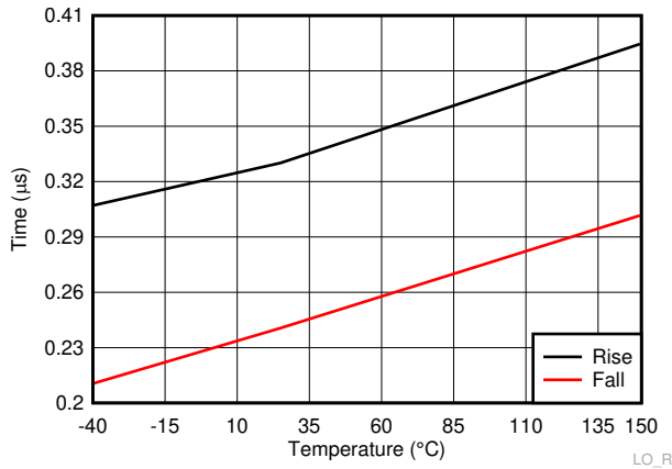
A. C_L=100nF Figure 6-21. LO Rise andamp; Fall Time
