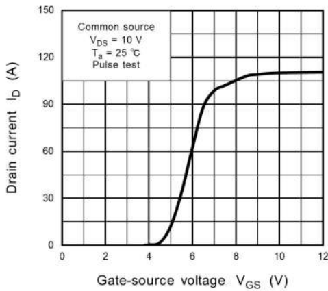
Fig. 8.3 I_D - V_{GS}
