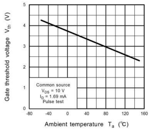
Fig. 8.10 V_{th} - T_a
