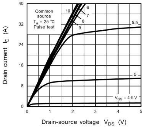
Fig. 8.1 I_D - V_{DS}
