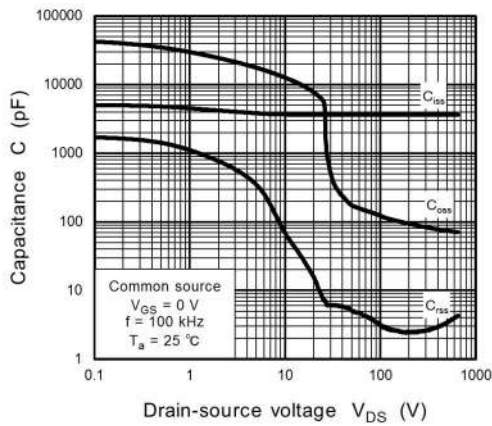
Fig. 8.9 C - V_{DS}
