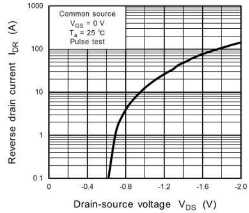
Fig. 8.8 I_{DR} - V_{DS}
