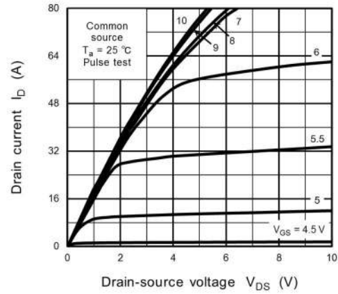
Fig. 8.2 I_D - V_{DS}
