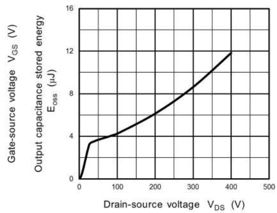
Fig. 8.12 E_{OSS} - V_{DS}
