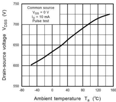
Fig. 8.5 V_{DSS} - T_a
