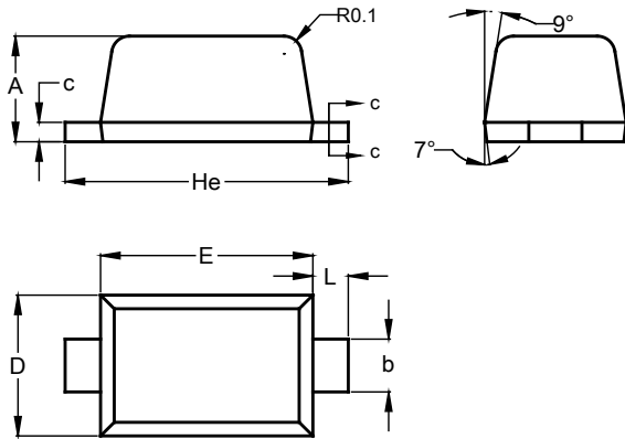
SOD523
