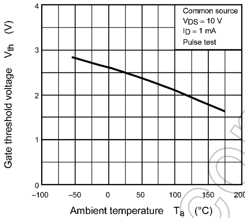
Fig. 9.9 V_{th} - T_a
