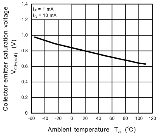
Fig. 11.9 V_{CE(sat)} - T_a
