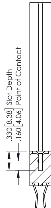
SECTION A-A
