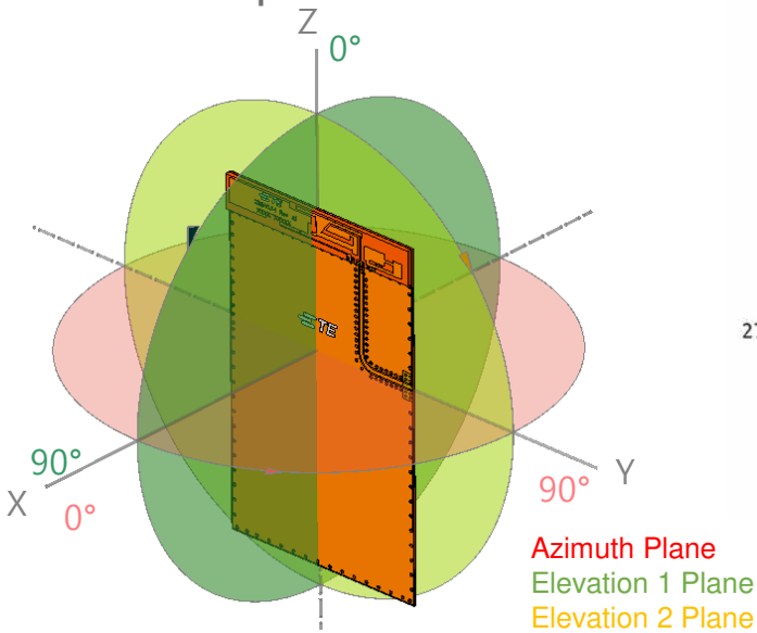
Elevation 1
