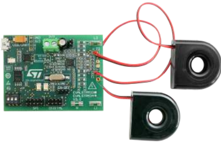
EVALSTPM34 board
