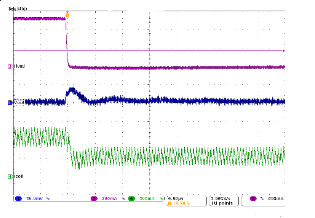
500 mA to 1 A, Falling edge
