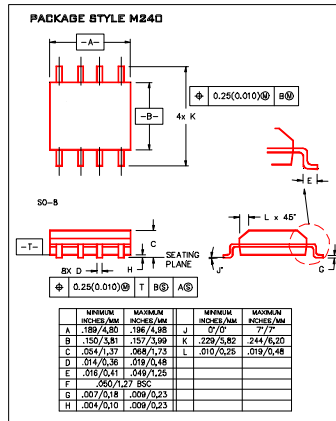
SO-8
