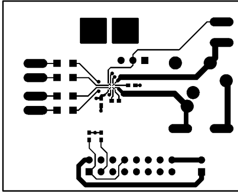
Figure 30. Top Layer
