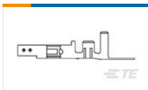
TE Part #2238017-1 VAL-U-LOK SKT BR SN 18-22AWG
