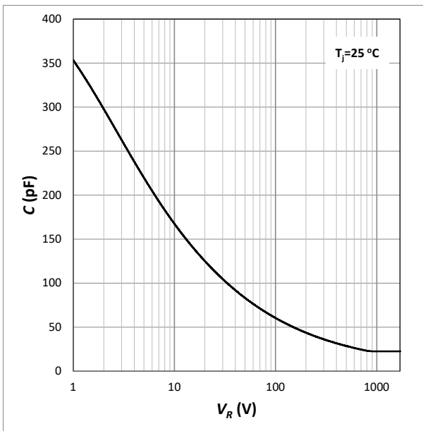
Fig. 5 Capacitance
