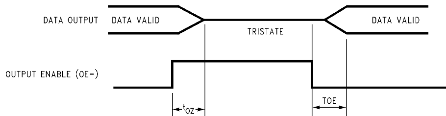
Data Output Enable
