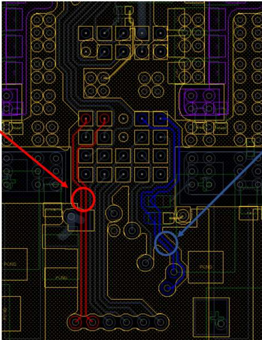
Figure 33 : VSense Traces
