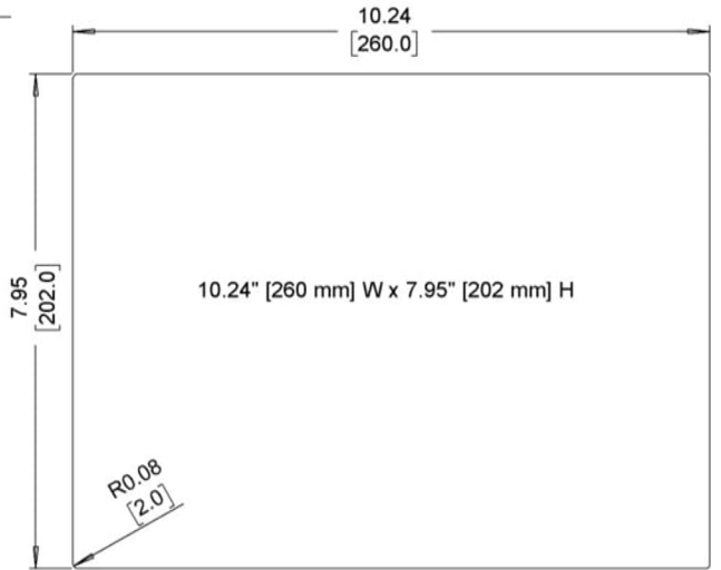
Cutout Dimensions
