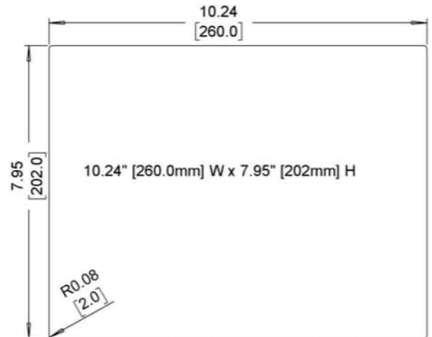
Cutout Dimensions
