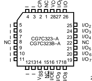
JEDEC PLCC [1] Top View
