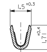
断面 A-A SECT. A-A
