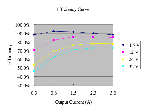
Vo=1.8 V
