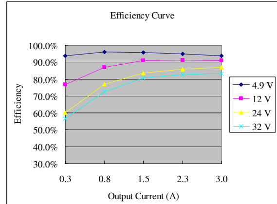
Vo=3.3 V
