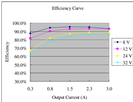
Vo=5.0 V
