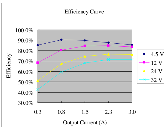
Vo=1.5 V
