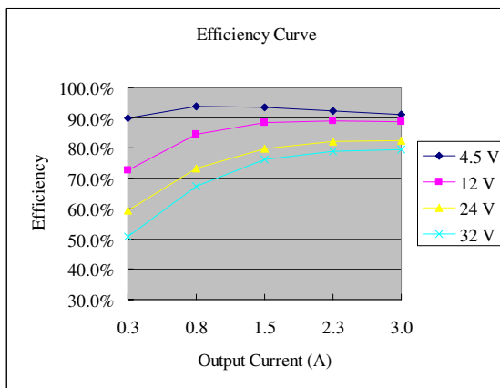
Vo=2.5 V
