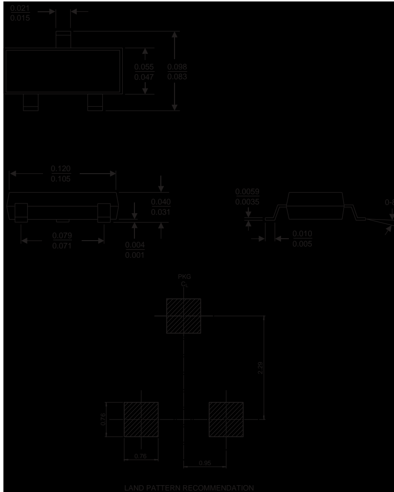
SOT-23 Package Dimensions FS Pkg Code AU
