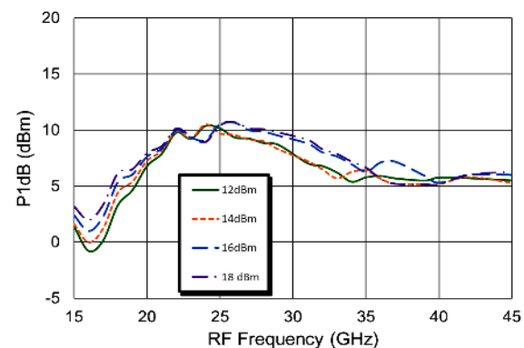
P1dB vs. LO power
