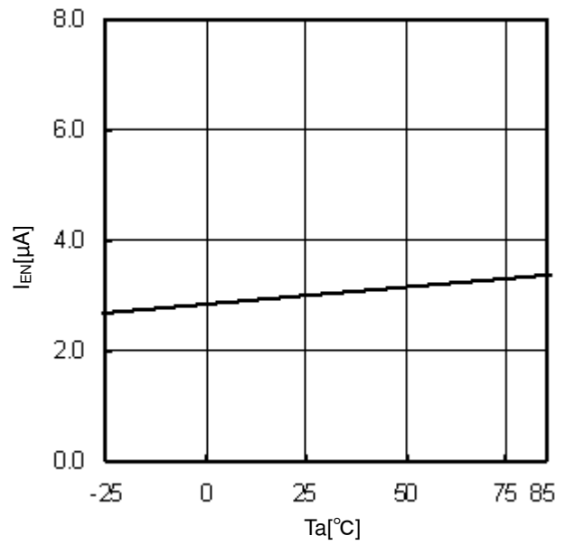
Fig.12 T_a - I_{EN}
