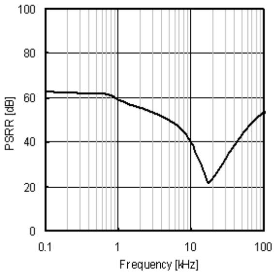
Fig.21 PSRR( I_o=0mA )
