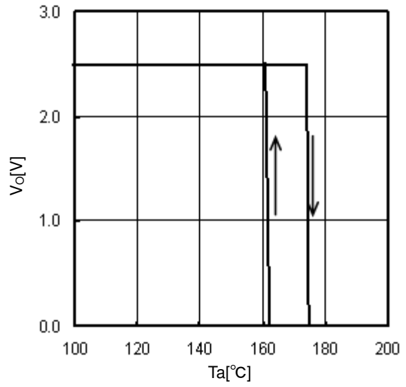
Fig.16 TSD ( I_o=0mA )
