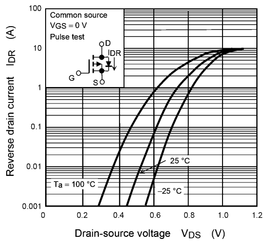
Fig. 8.9 I_{DR} - V_{DS}
