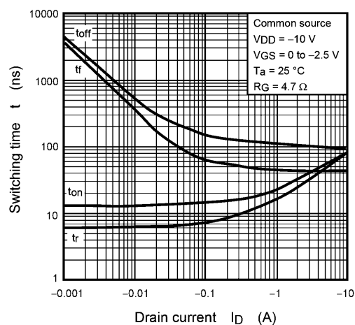
Fig. 8.11 t - I_D
