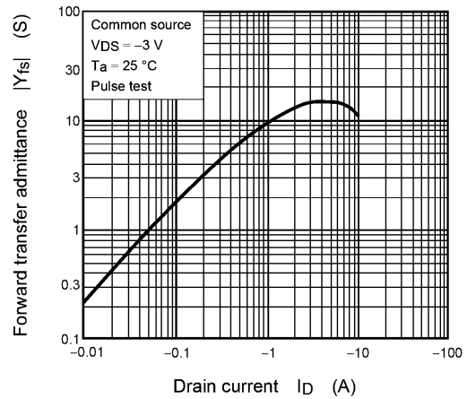
Fig. 8.8 |Y_{fs}| - I_D
