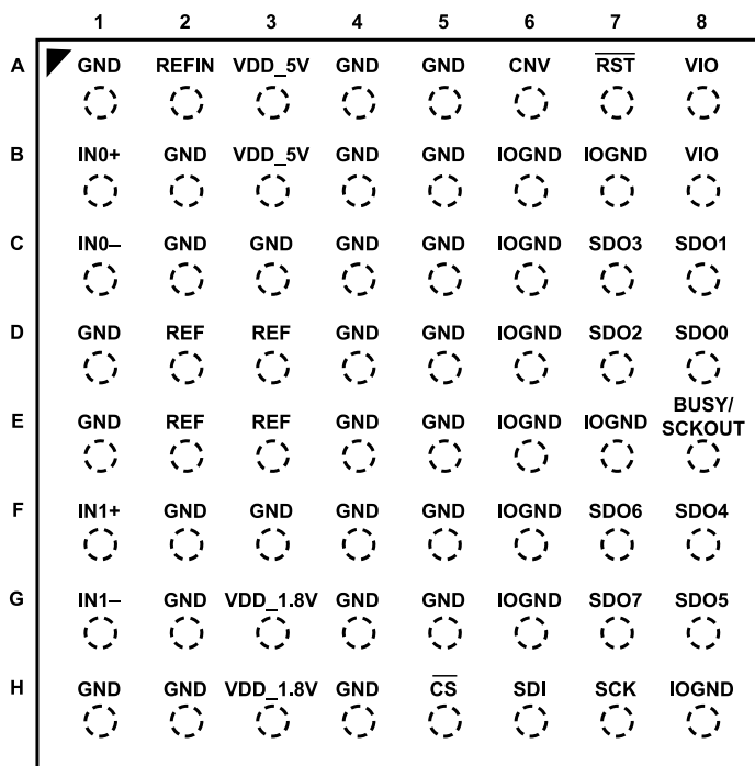
AD4630-24/AD4632-24 TOP VIEW
