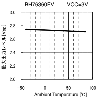
Fig.28 Vom vs. Ambient Temperature
