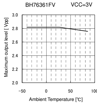
Fig.30 Vom vs. Ambient Temperature
