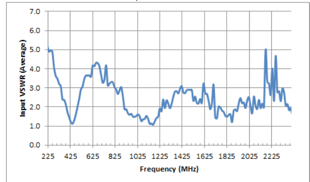
Input VSWR
