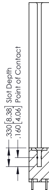
SECTION A-A
