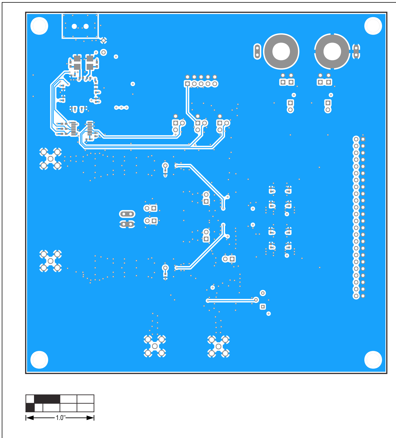
MAX19505/MAX19506/MAX19507 EV Kit PCB Layout—Bottom Layer
