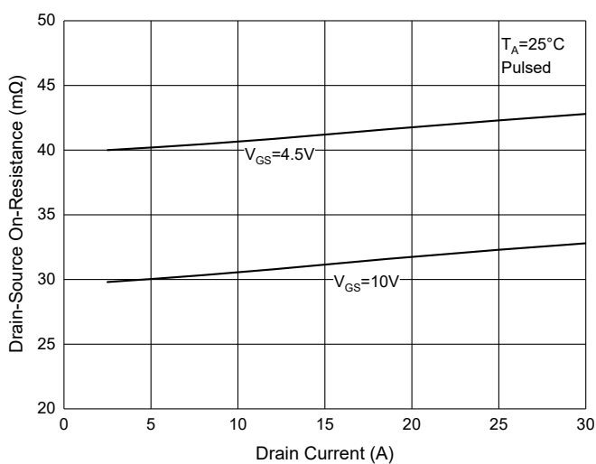
Fig. 5 - R_{DS(ON)} - I_D
