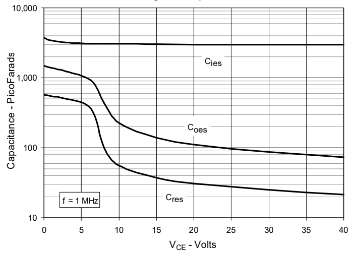
Fig. 10. Capacitance
