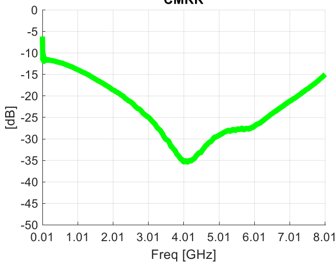
CMRR
