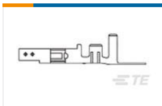
TE Part #794956-1 VAL-U-LOK SKT BR SN 22-18AWG
