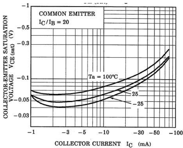
Fig. 10.21 RN2903 V_{CE(sat)} - I_C
